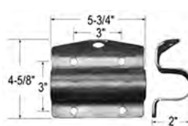
1. FRUDCF2139-1 Lock rod guide
