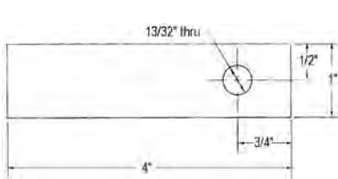
1. PEN25-03
