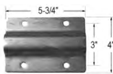
1. FRUDCF2137-1 Lock rod guide
